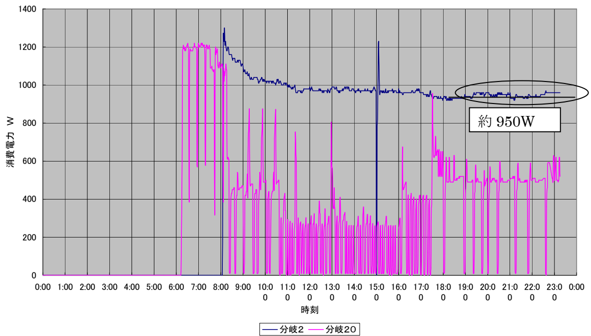
居間・キッチンエアコン消費電力2010/2/6
