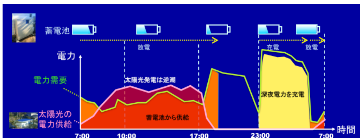
図 4-4 蓄電池システムの充放電制御例（逆潮優先方式）
