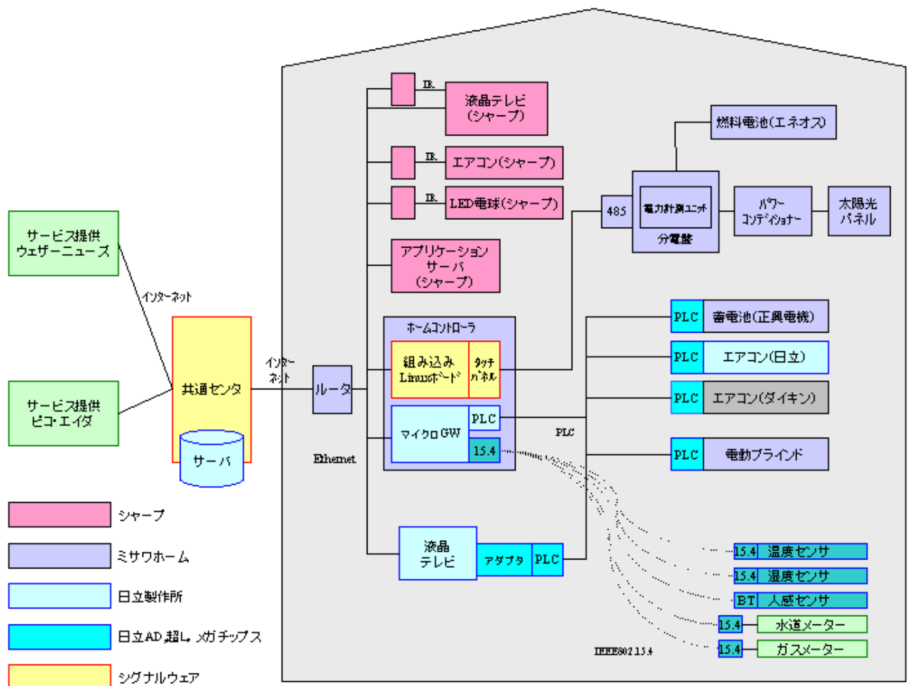
図 4-26 システム全体のアーキテクチャと主な分担
