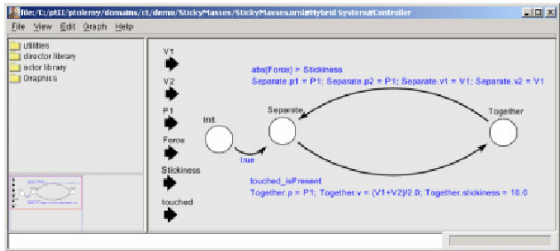
図 3.3 Vergil の状態遷移図の例
