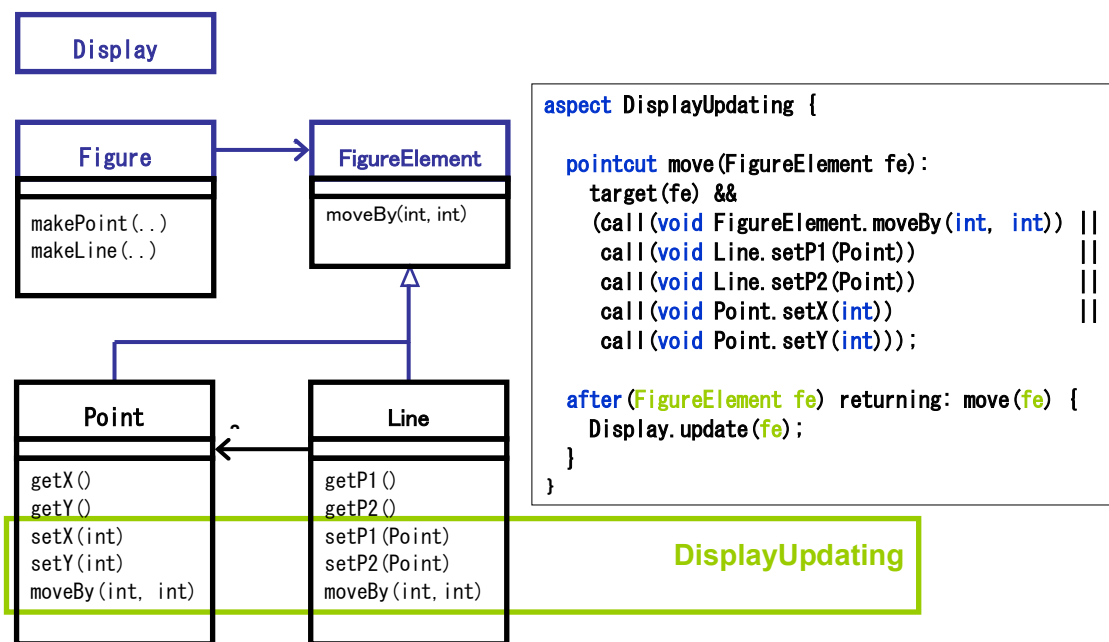
図 3.5 Aspect/J による図形要素と画面の再描画の例
