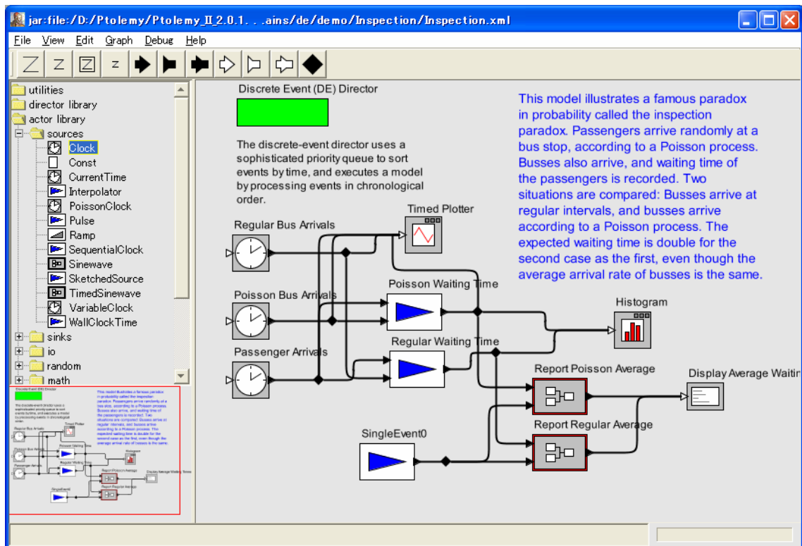
図 3.2 Vergil のバス停における待ち行列のシミュレーション例
