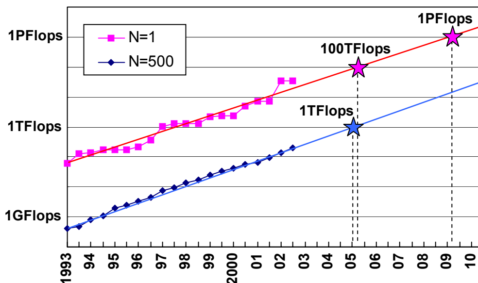
図 2.2 Top 500 の性能トレンド
