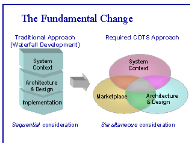
図 3.8 CBS の開発手法のアプローチ
