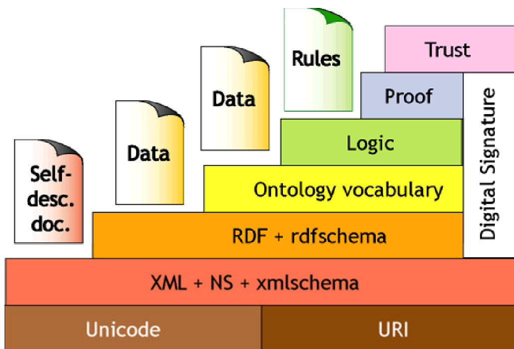
図 3.6 Semantic Web のアーキテクチャ
