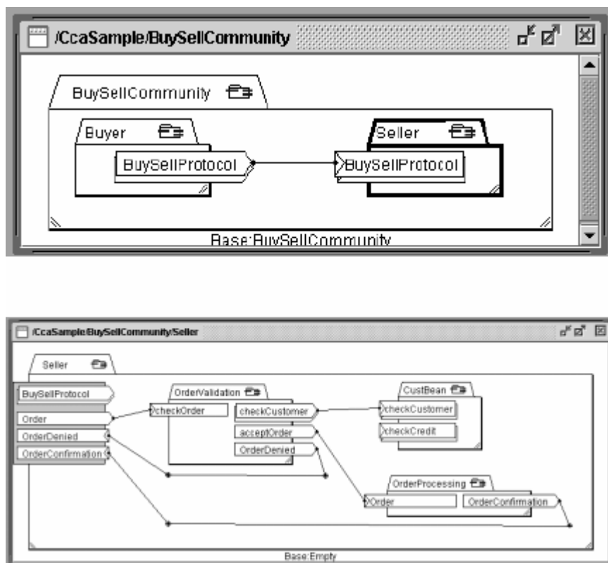
図 3.4 EDOC の CCA(Component Collaboration Architecture)による販売の例
