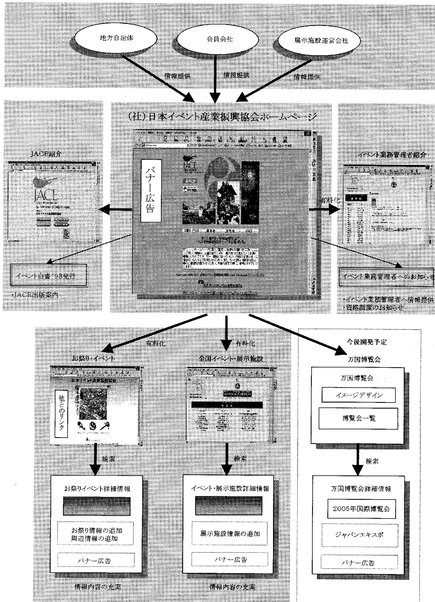
図3-19: 今後の事業展開図
