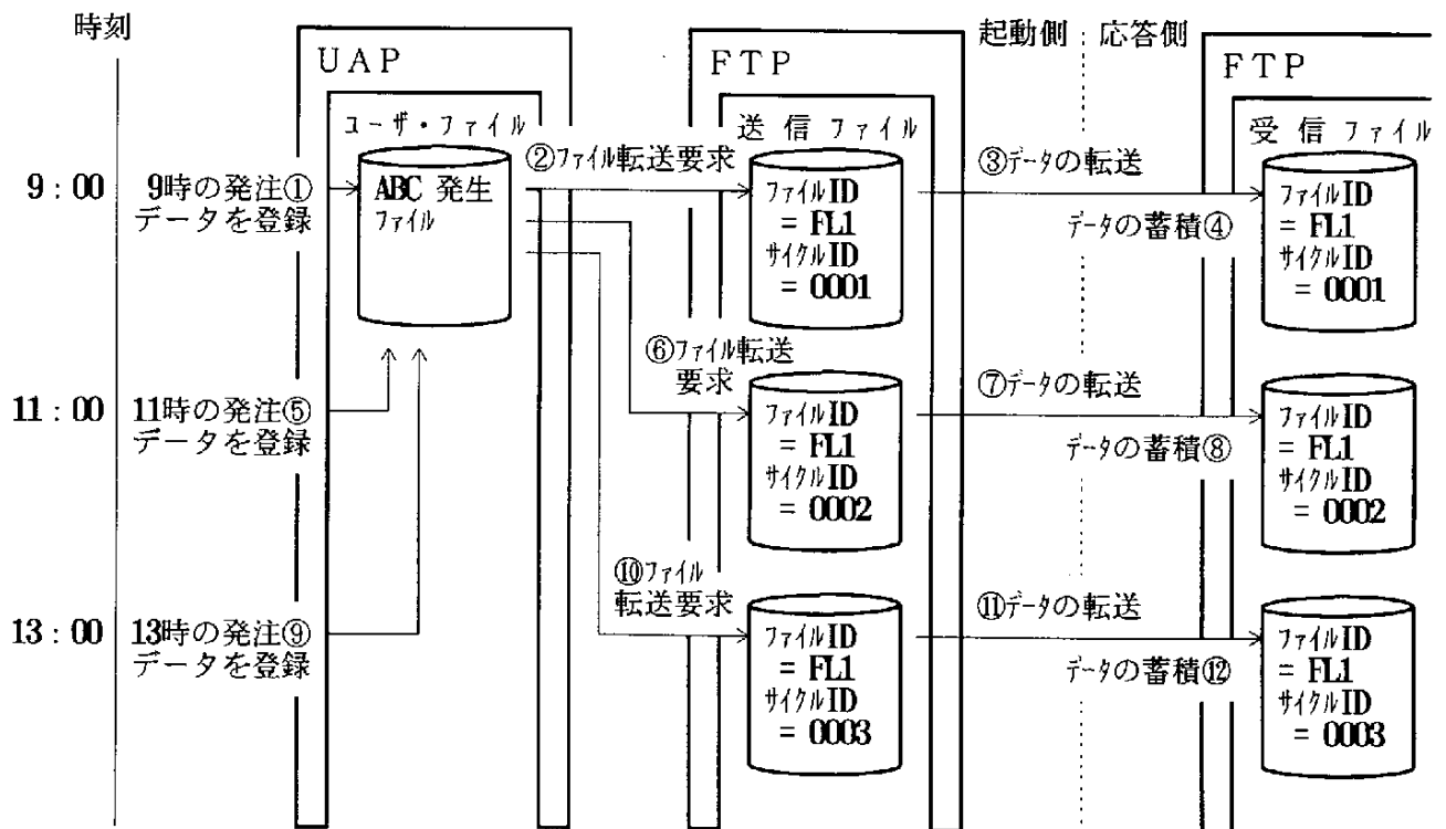
図3-1 サイクルID自動採番の事例
