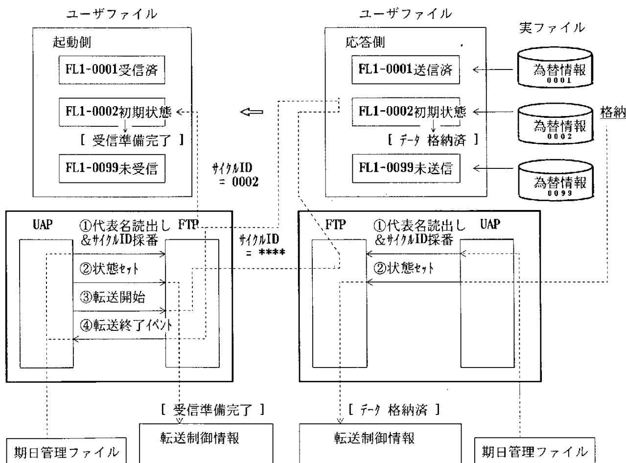
図3-4 代表名によるファイル読出しの利用事例
