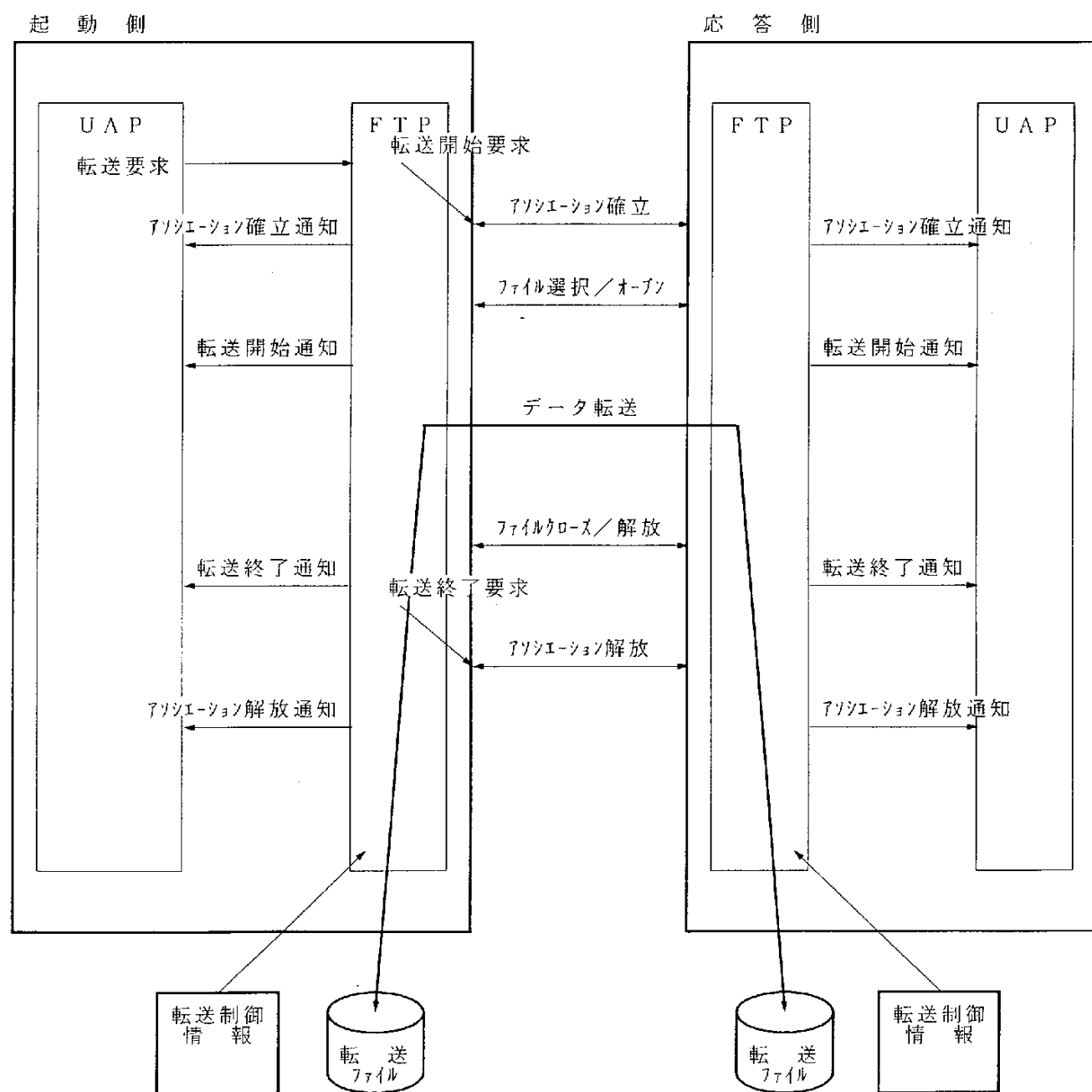
図3-1 ファイル転送基本機能
