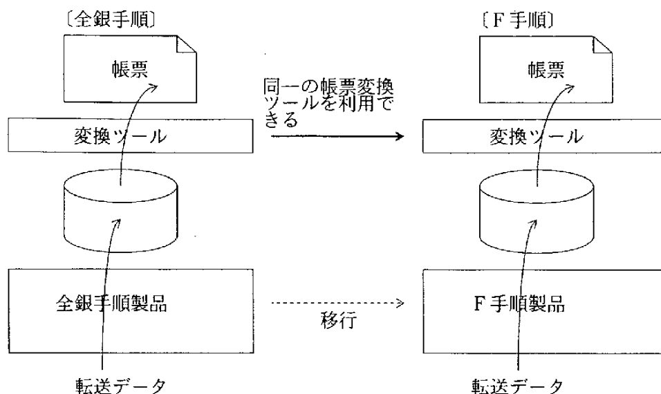
図6-6 ディレイド変換によるデータ交換フォーマットの移行
