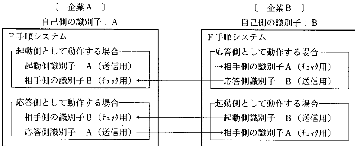
図 2 - 3 起動側識別子と応答側識別子の送信
