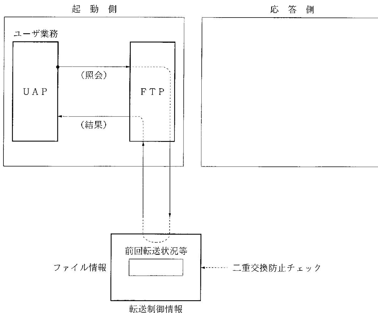
図3-9 起動側での二重交換防止チェック
