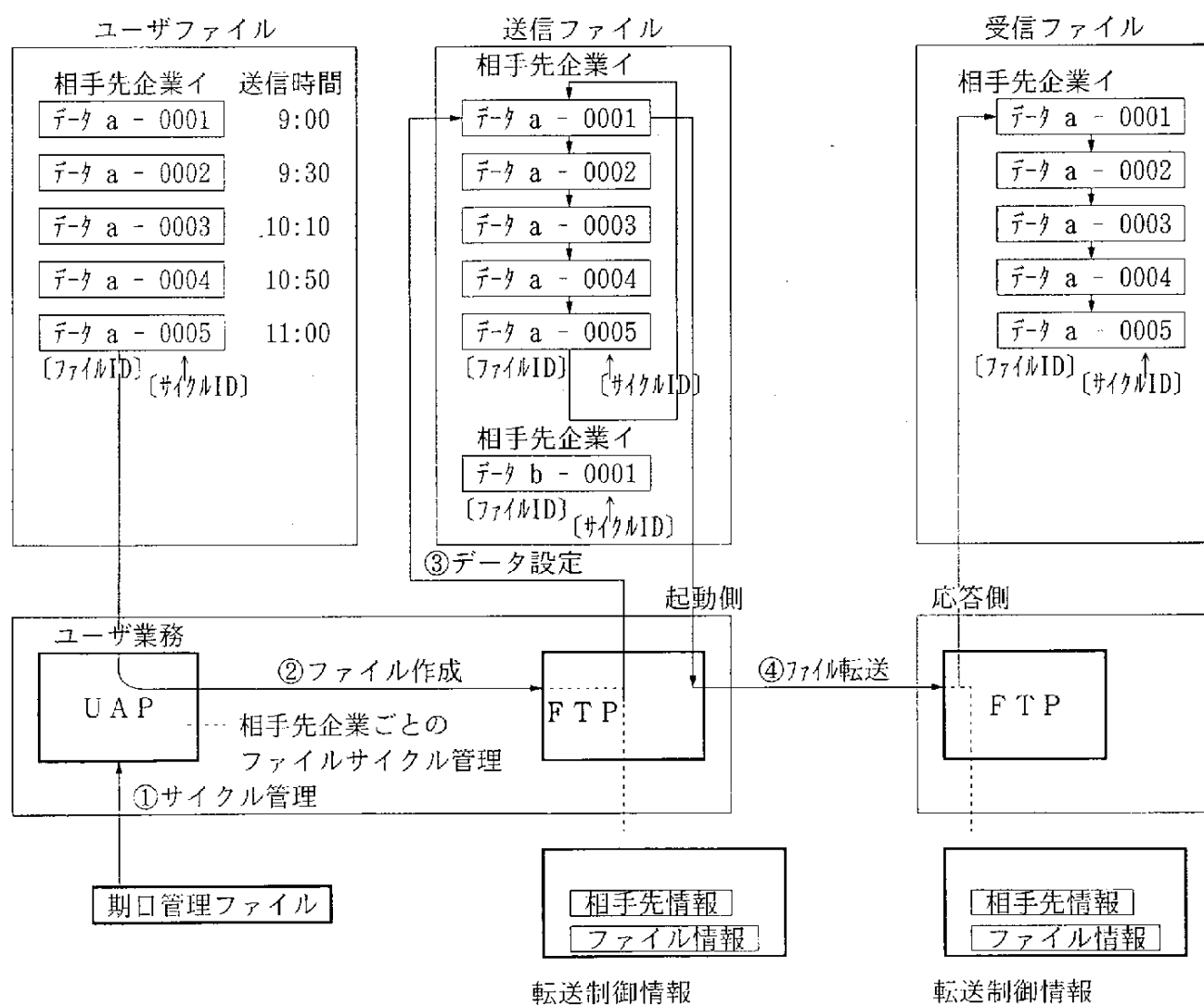
図3-8 サイクル管理
