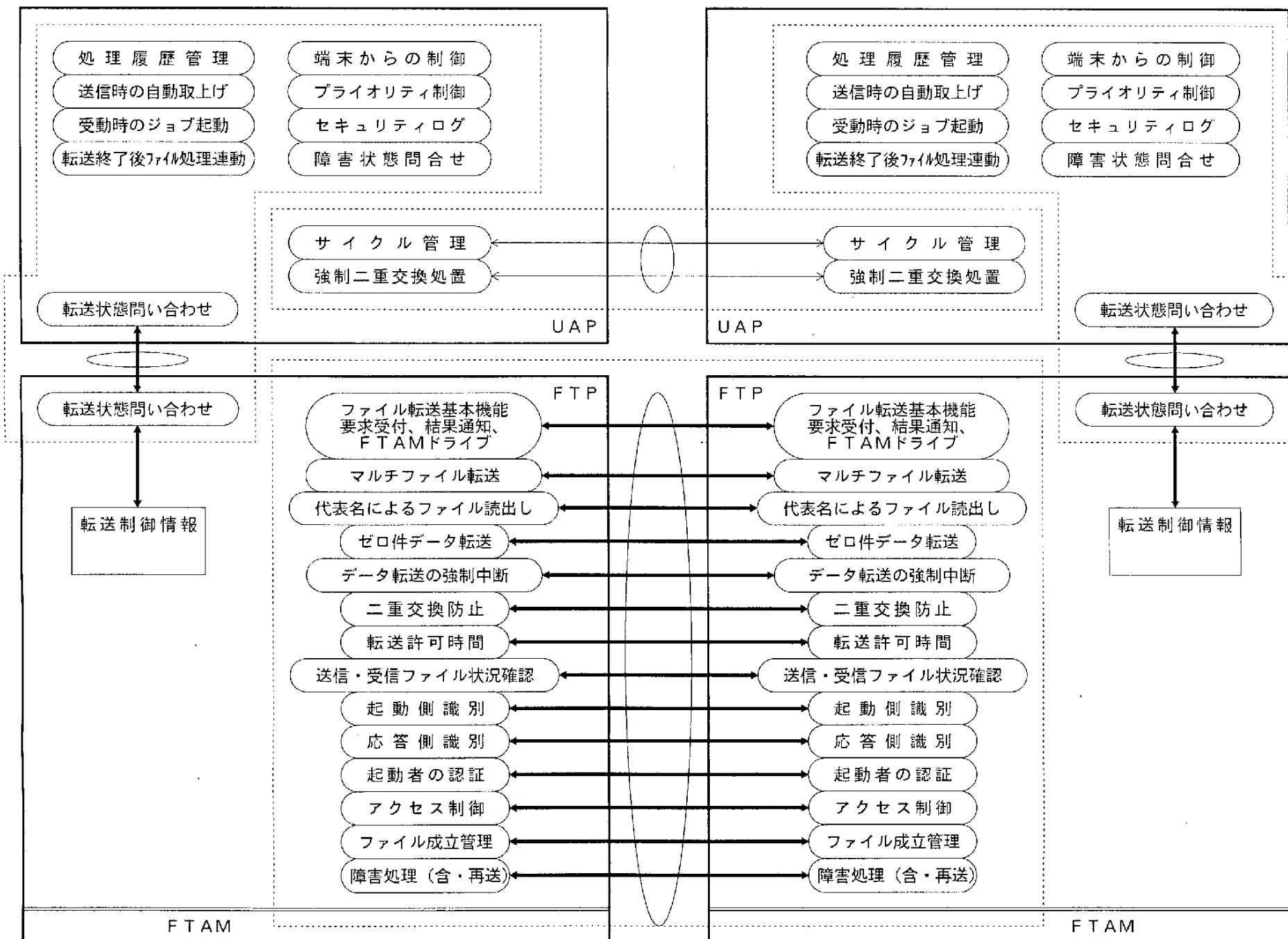
図2-3 F手順の機能構造
