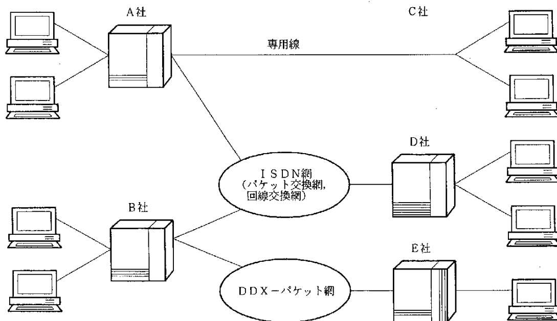
F手順回線利用形態の例
