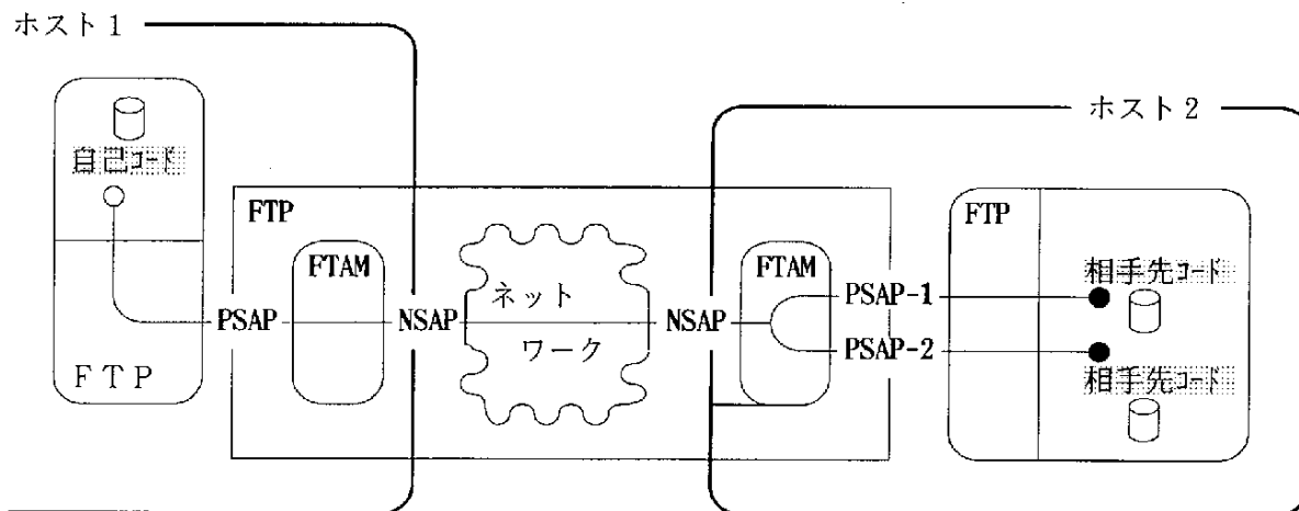
図2—4 ユーザシステム間接続のネットワーク構成定義例
