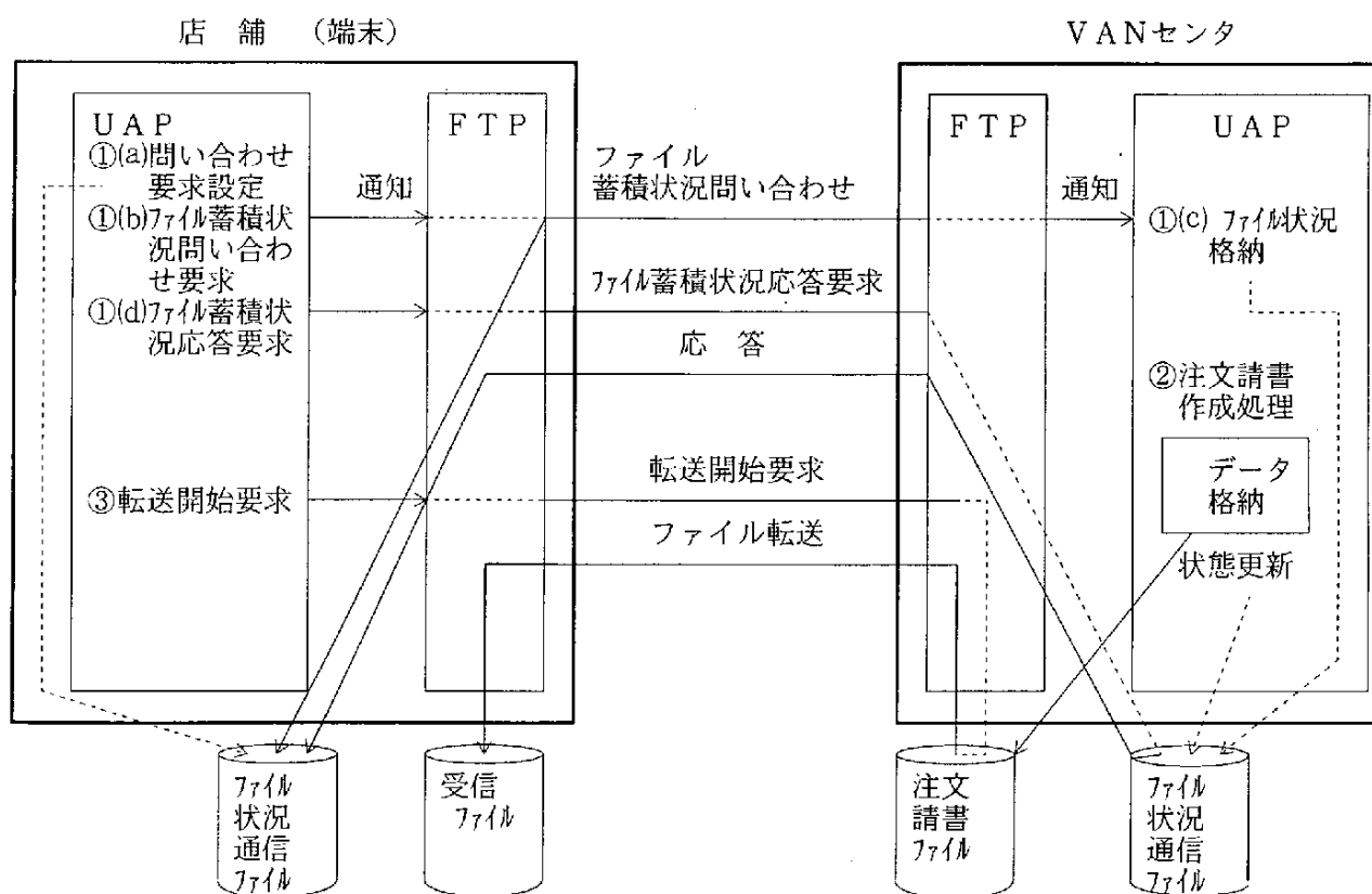
図3－7 ファイル蓄積状況問い合わせに関する利用事例
