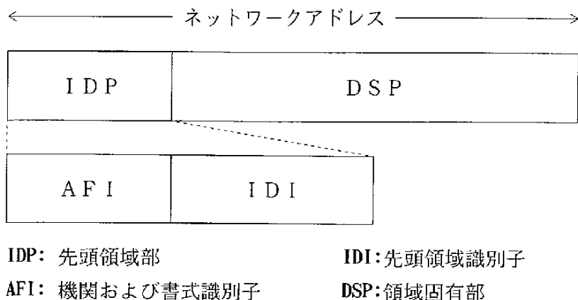
図1 ネットワークアドレスの構造
