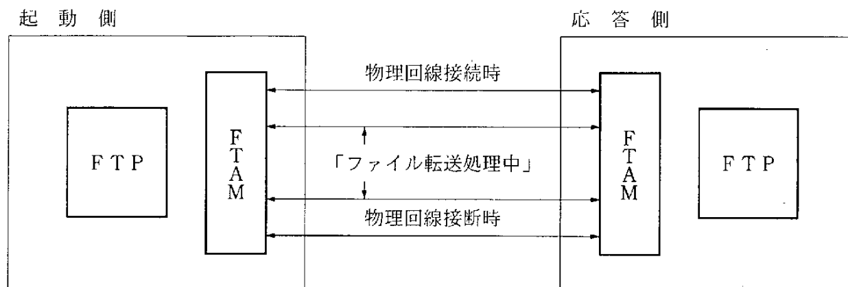
図3-31 障害状態
