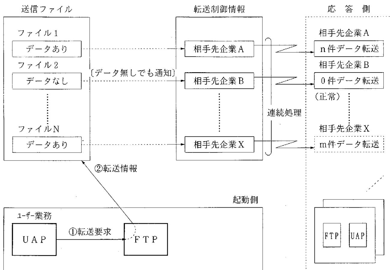
図3-6 ゼロ件データ転送
