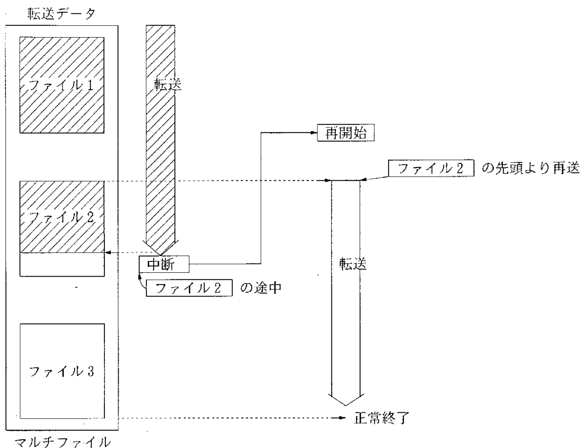
図3-4 マルチファイル転送における再送処理
