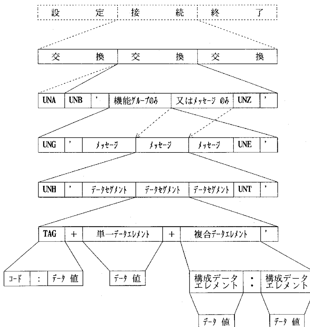
図4-3 EDIFACTによるデータ交換フォーマットの階層
