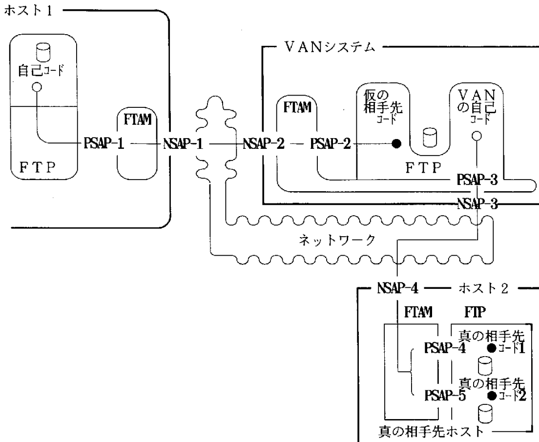
図2-5 VAN利用のネットワーク構成定義例
