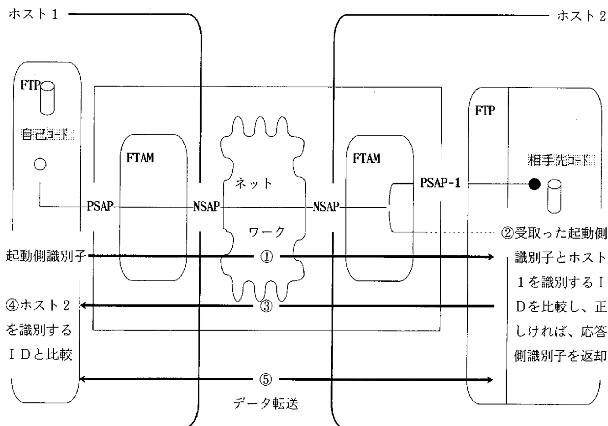
図2-6 起動側識別子と応答側識別子の利用動作の例
