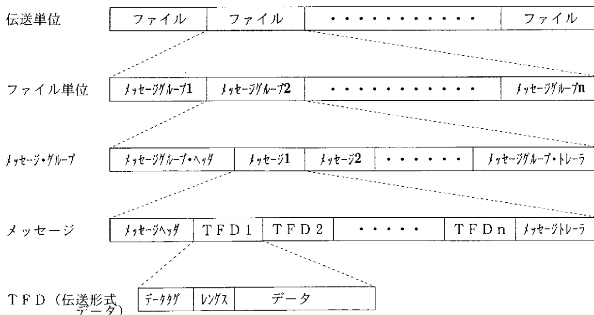
図4-1 CIIシンタックスルールによるデータ交換フォーマットの階層
