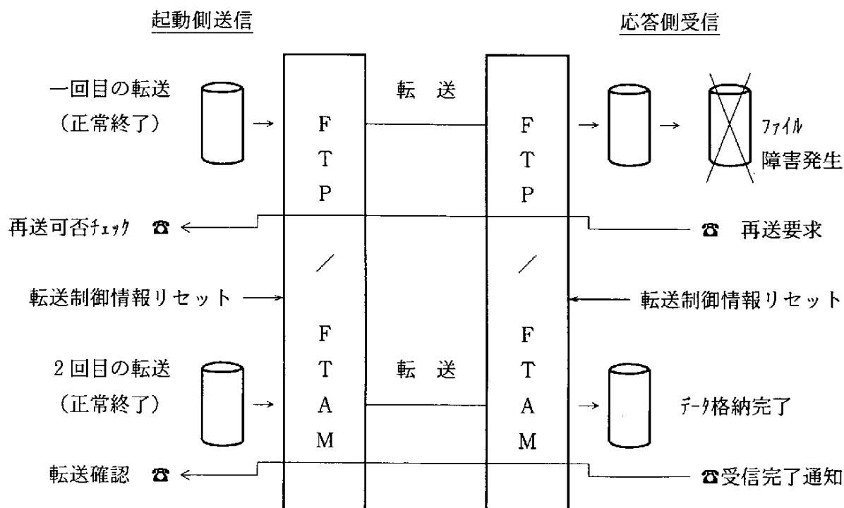
図3-9 強制二重交換処置手順
