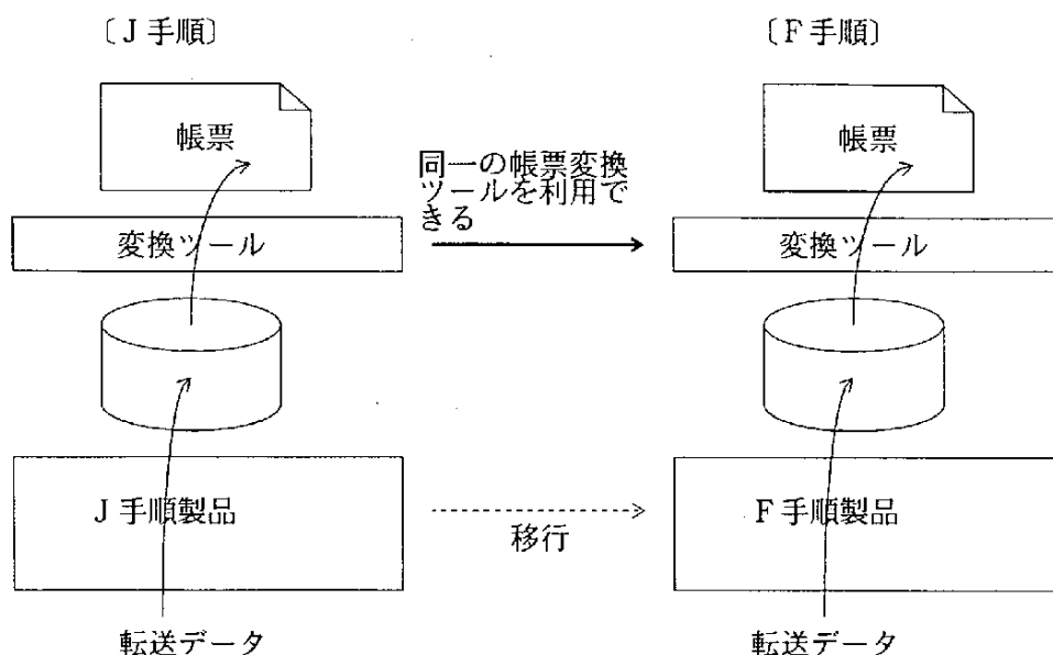
図 6-3 ディレイド変換によるデータ交換フォーマットの移行
