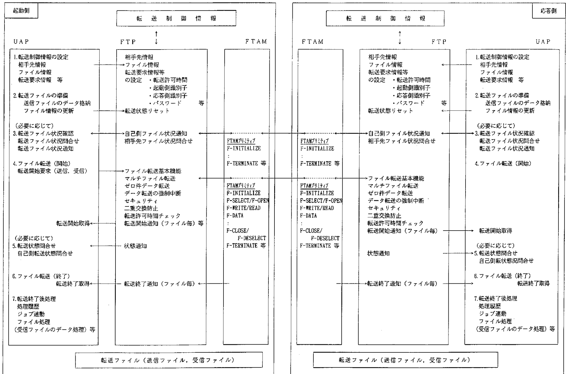
図 2-4 代表的な基本シーケンス
