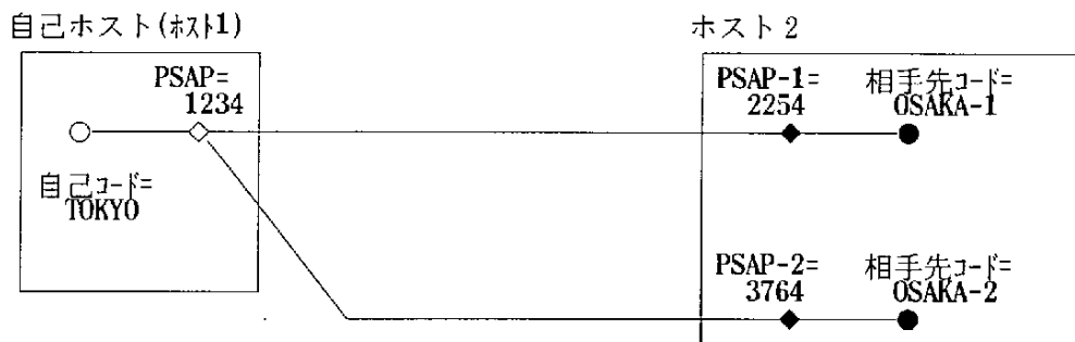
図2—4 ユーザシステム間接続のネットワーク構成定義例
