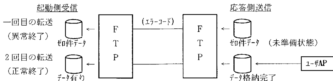
図3-10 データ準備遅延時の処理
