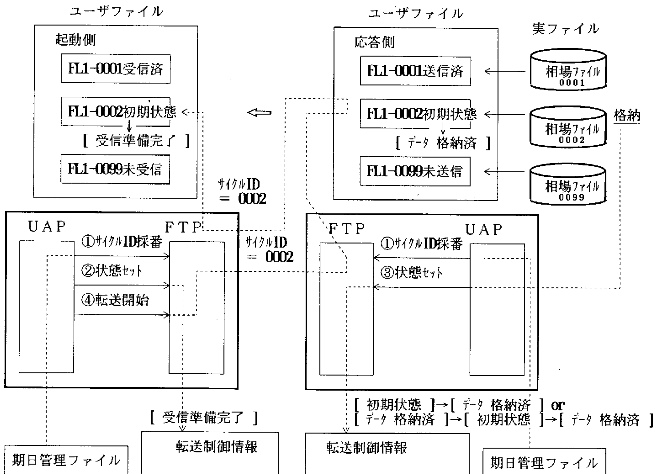
図３－３ サイクル管理に関する利用事例－２
