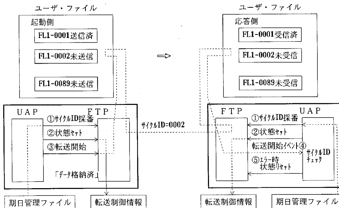
図3－2 サイクル管理に関する利用事例－1
