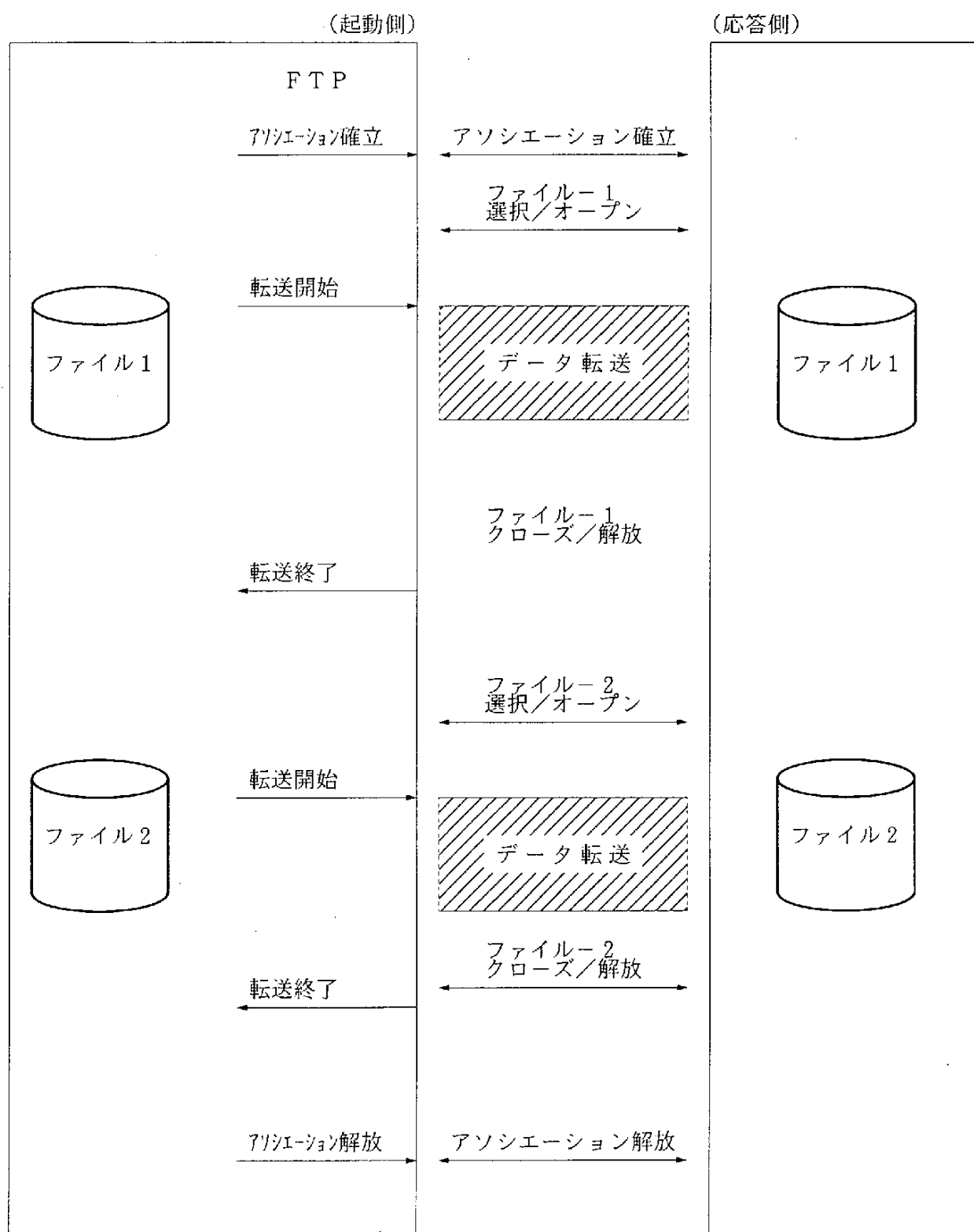
図3-3 マルチファイル転送処理手順
