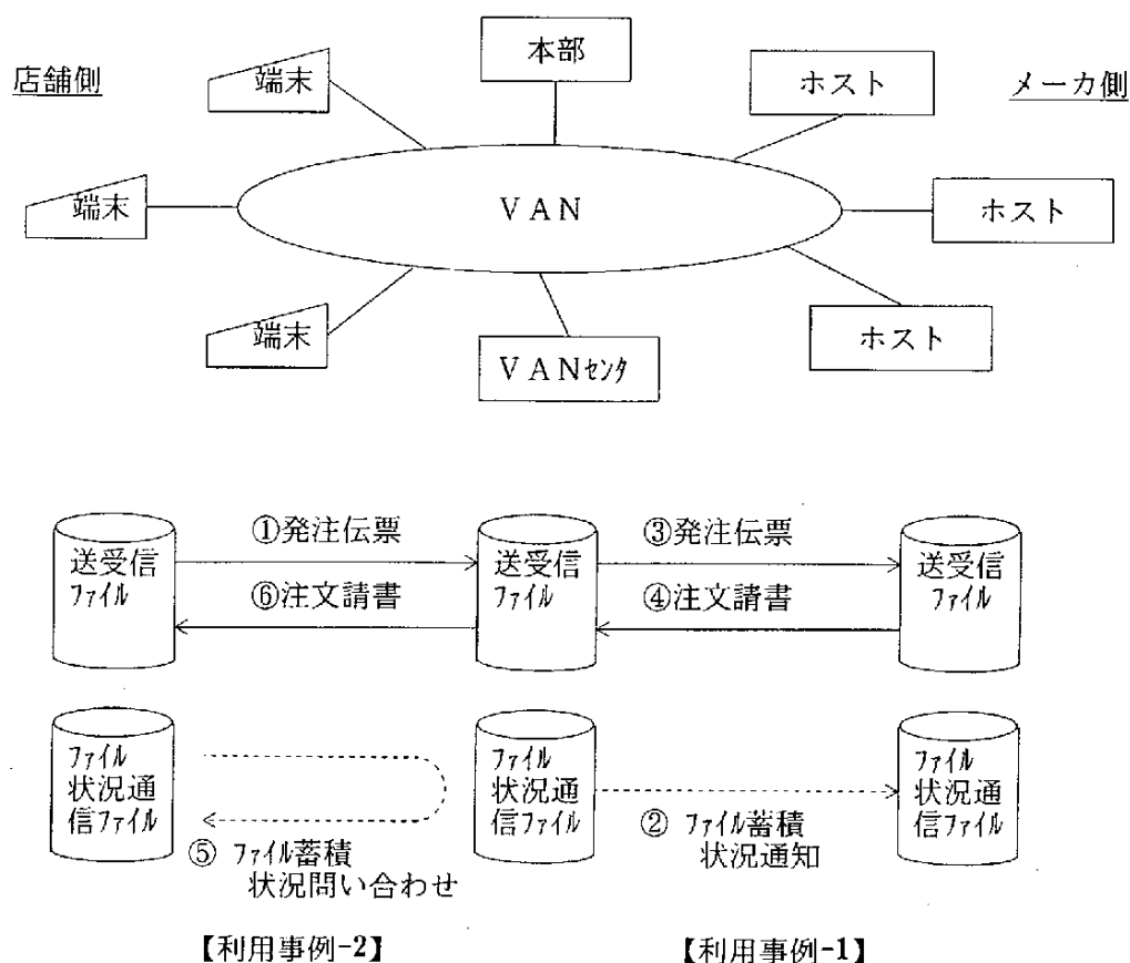
図3-5 受発注VANでの受発注データの蓄積交換処理に関する利用事例
