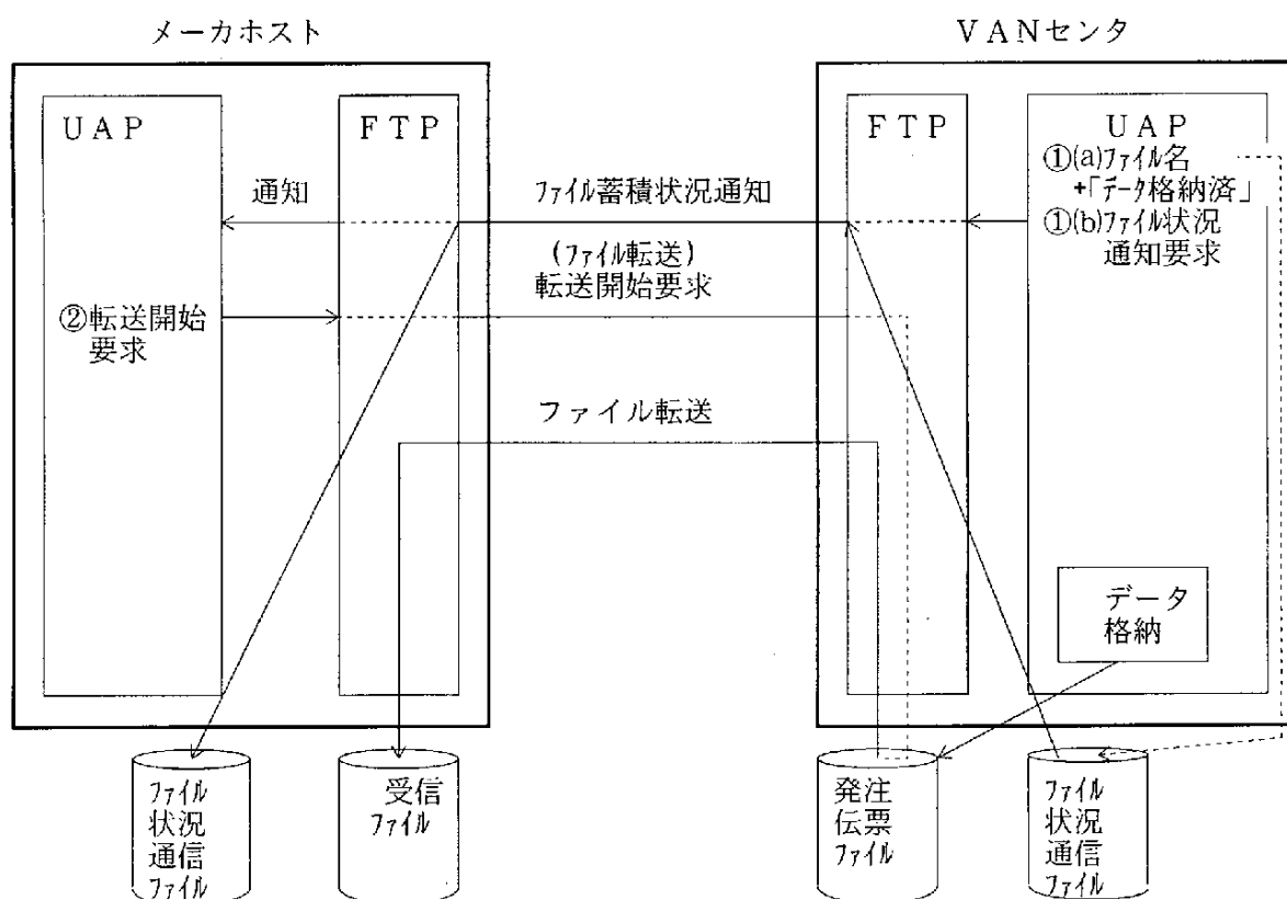
図３－６ ファイル蓄積状況通知に関する利用事例
