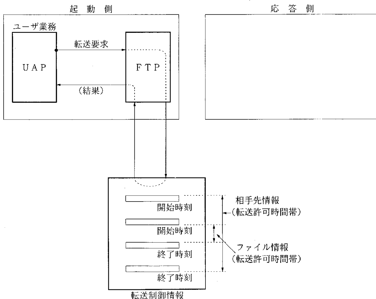
図3-12 起動側での転送許可時刻設定
