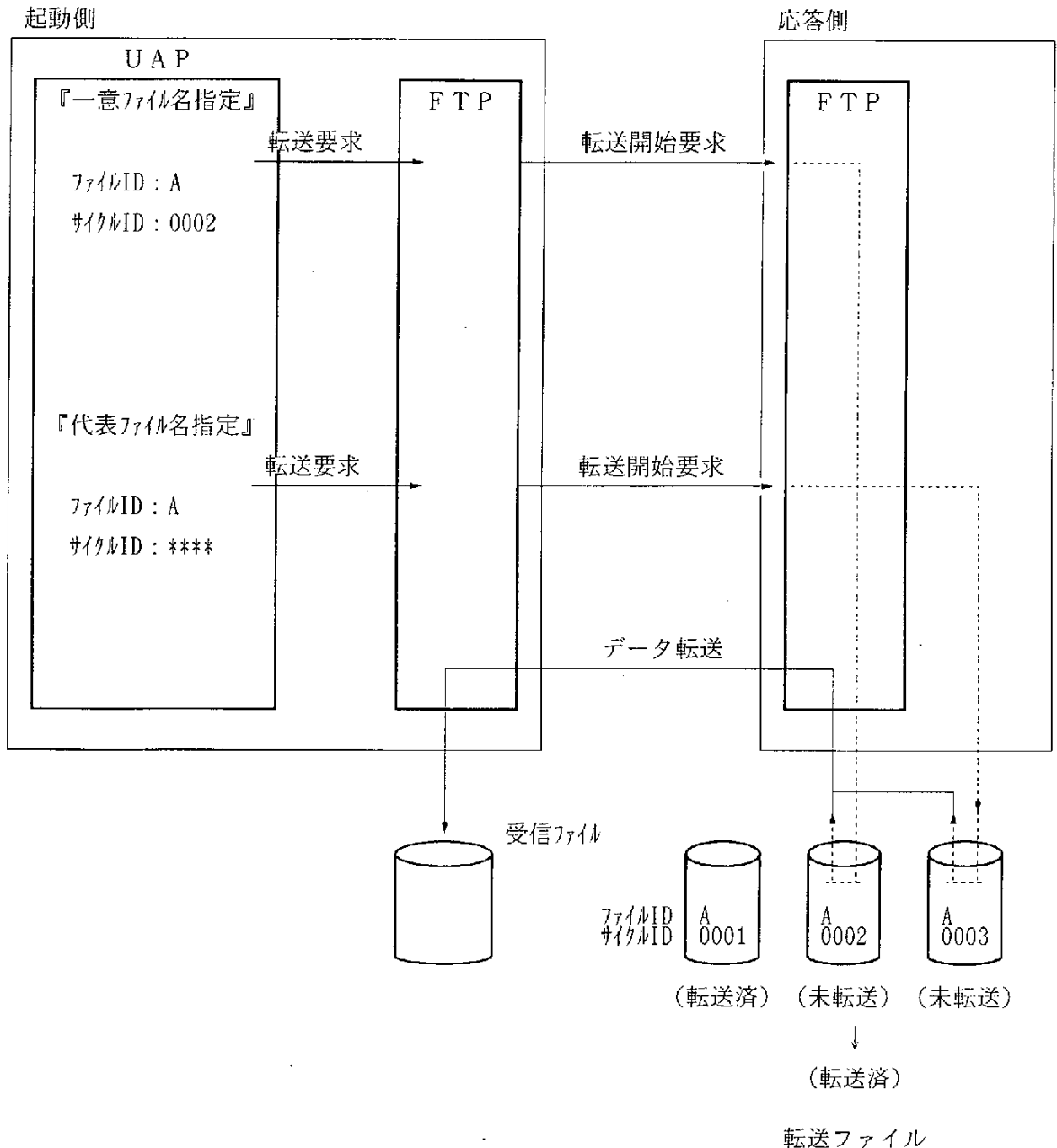
図3-5 代表名によるファイル読出し
