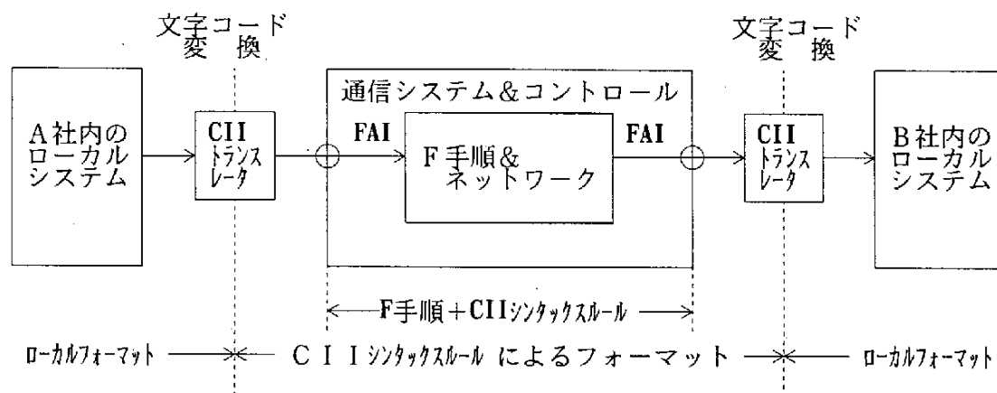
図4-2 トランスレータを活用したE D I
