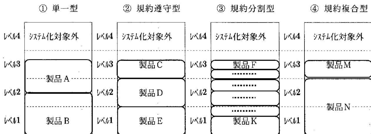
図 1 - 3 E D I 規約と F 手順製品サポート範囲の関係
