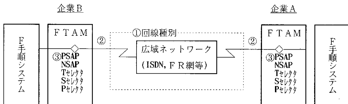
図2-1 F T A M環境
