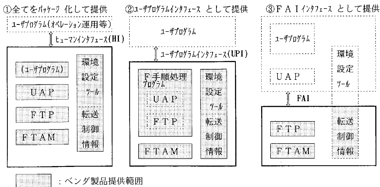
図1-6 製品の提供形態
